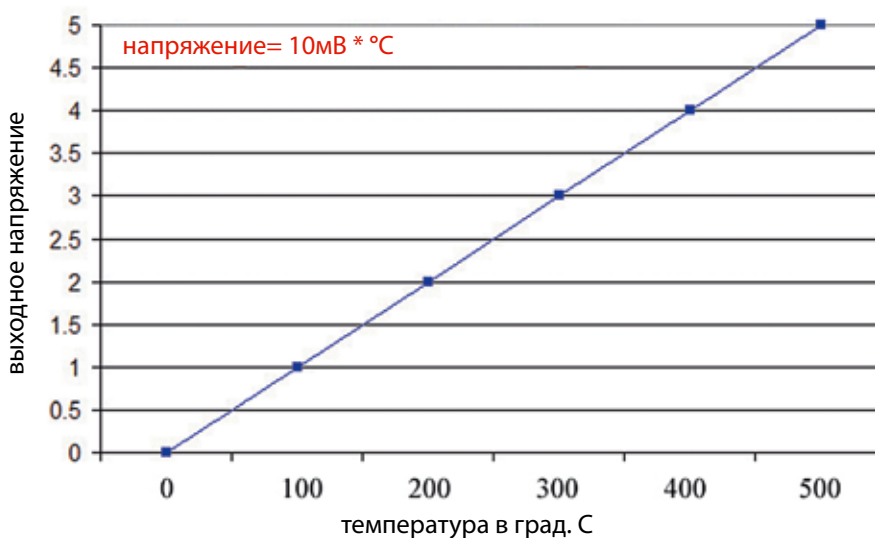
График: температура всасываемого воздуха относительно напряжения
